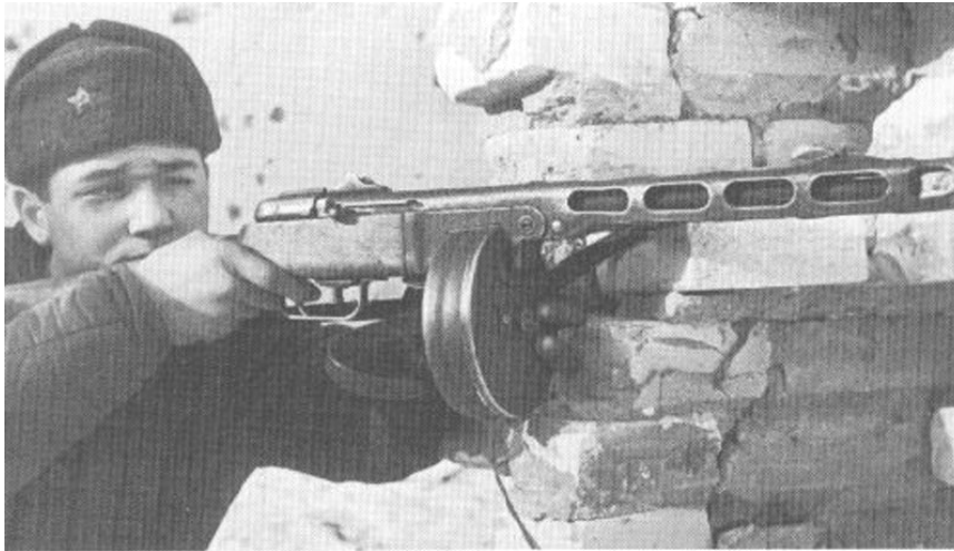
PPS-41 csigatáras géppisztoly
